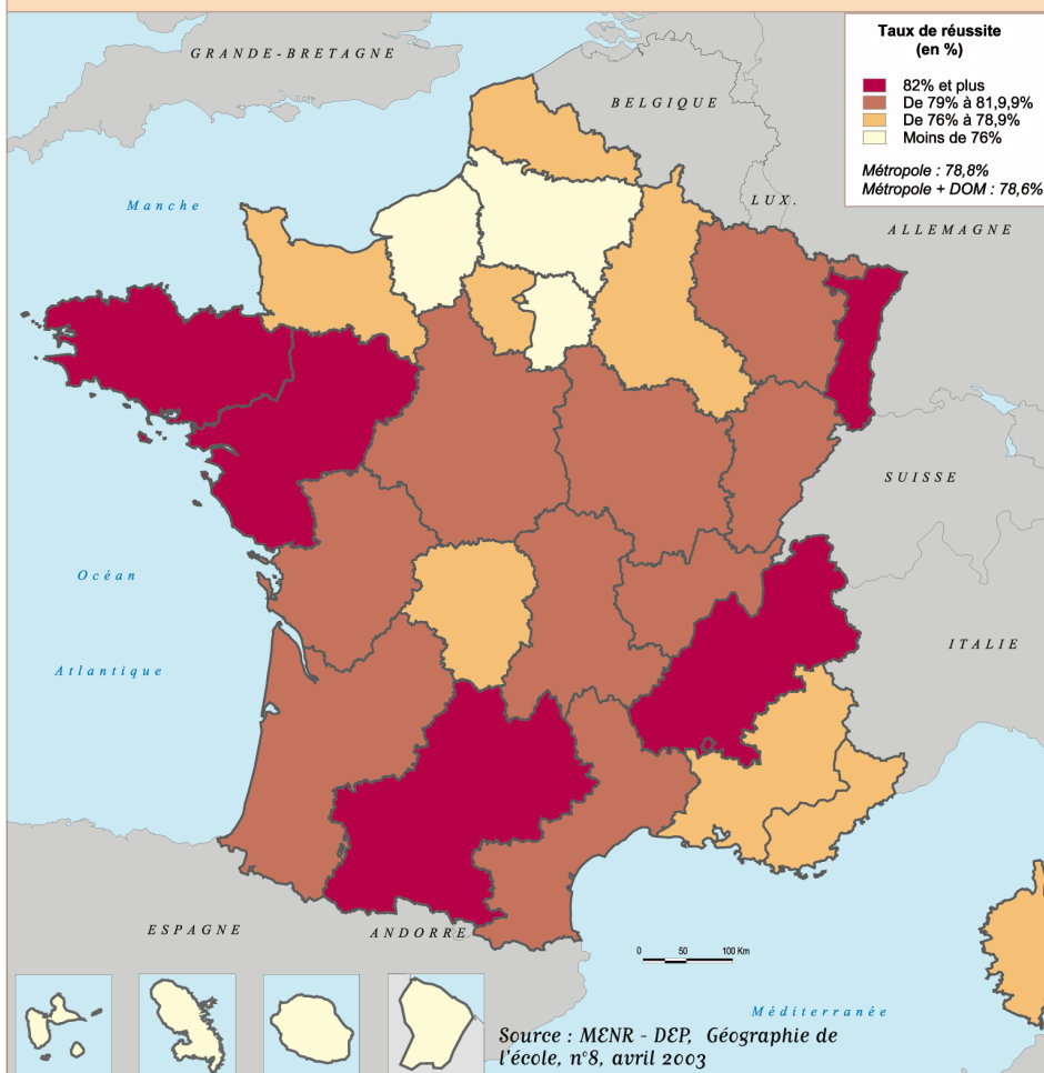
FIGURE 123 → Taux de réussite au Baccalauréat (en 2002) / France (régions)
